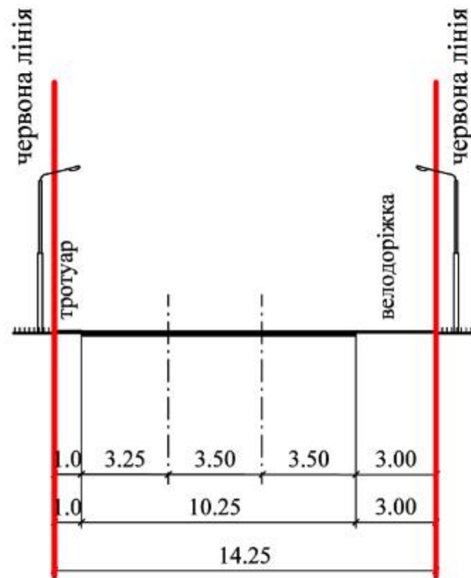
Розріз I-I
